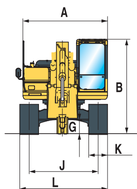
MONOBLOCK-AUSLEGER
